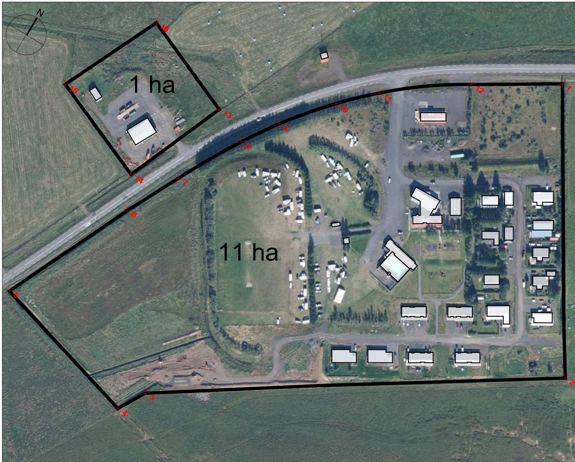
Upprétt loftmynd - yfirlitsuppráttur - mkv. 1:2.000 í A3
